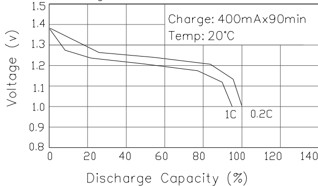
Discharge
